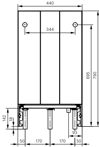
Vnitřná jednotka Pohľad spredu
