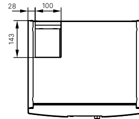
Vnitřná jednotka Pohľad zhora
