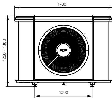
Vonkajší modul CHA Pohľad spredu
