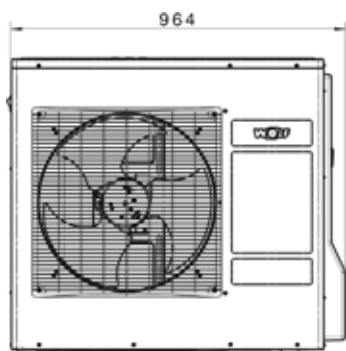
vonkajší jednotka BWL-1S(B)-05/07
